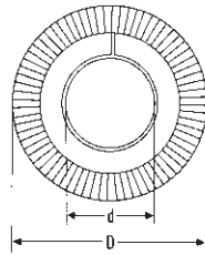
Ringbesatz außen/Ring outwards
